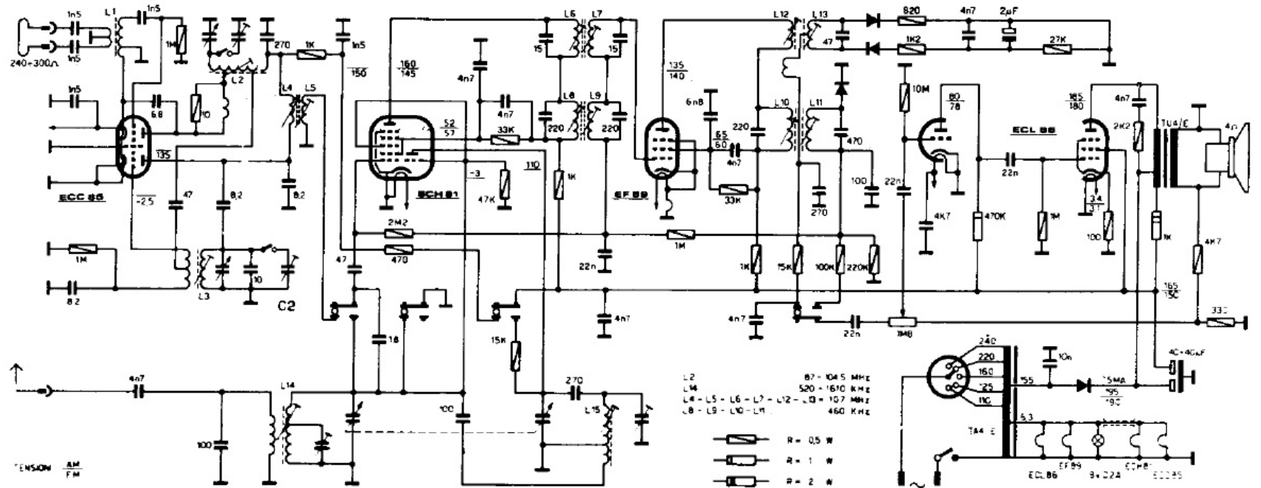
SCHEMA ELETTRICO DEL RADIORICEVITORE G.B.C. FM/1A II° DANDY
